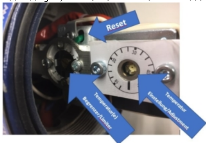
Abbildung 2) EX-Heizer Artikel-Nr. 1600210 Gehäuse/Casing blau/blue
