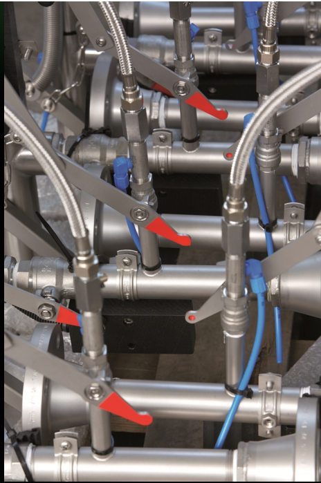
selbstentleerende Notdusche Detail Wasserauslass
